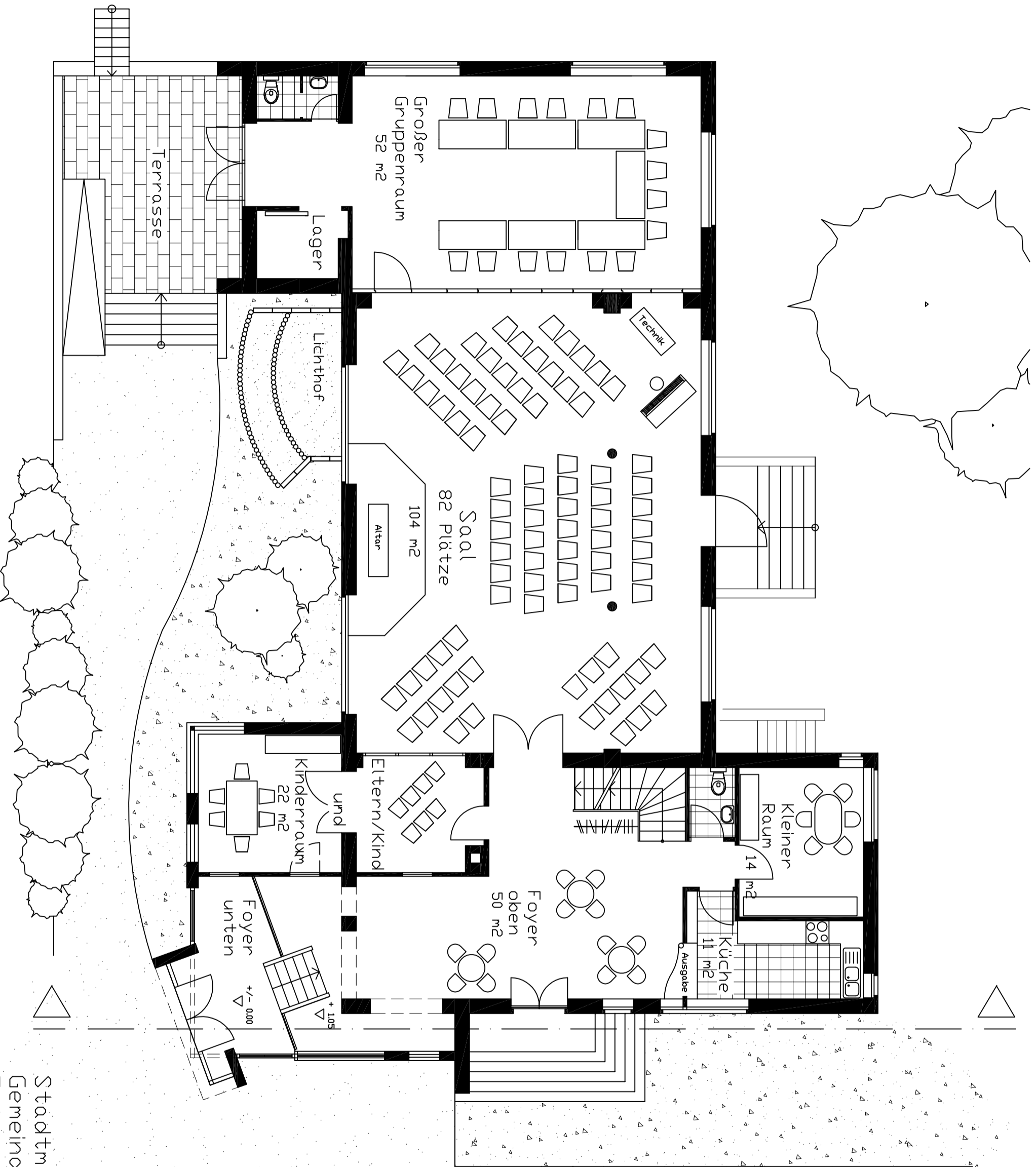
Grundriss Erdgeschoss
